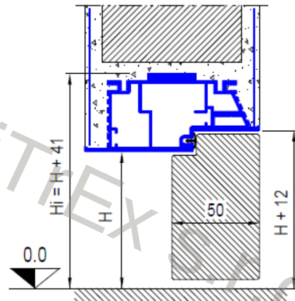
Zvislý rez
