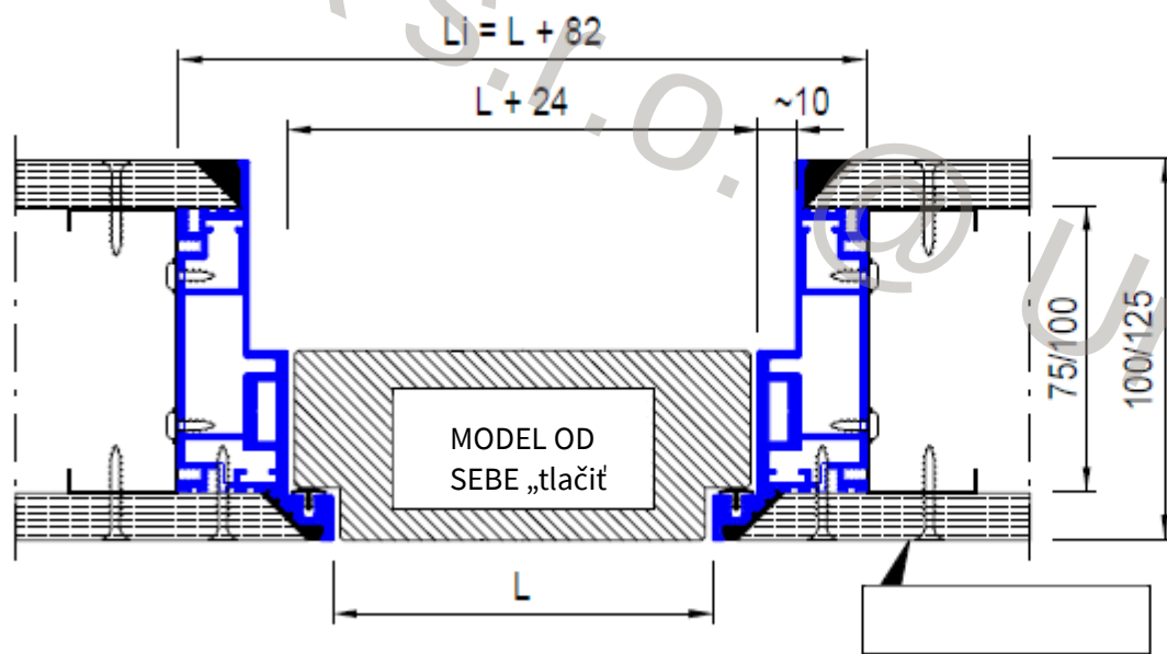
VODOROVNÝ REZ
