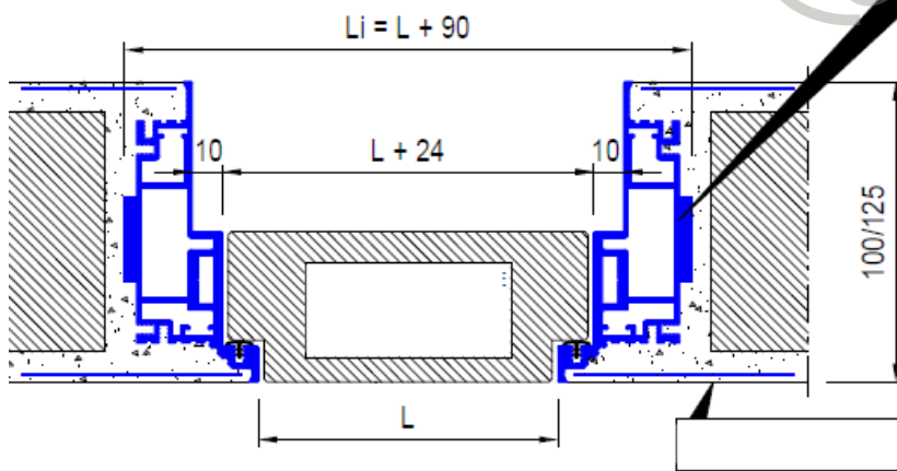
Vodorovný rez
